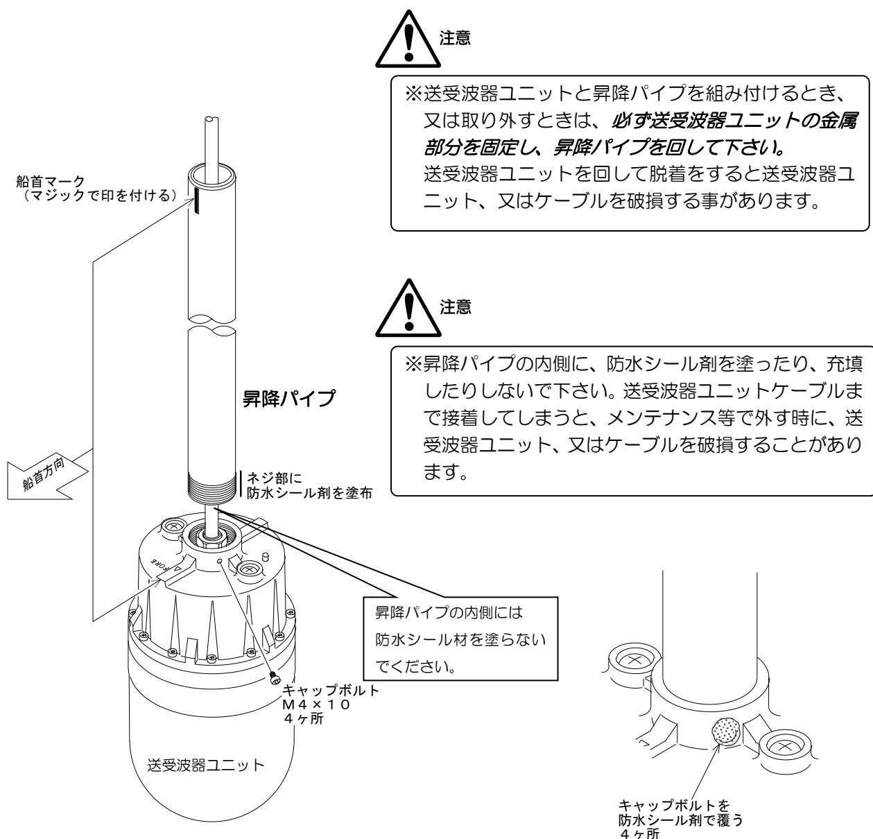
図 1.16 昇降装置部の組立要領-1
