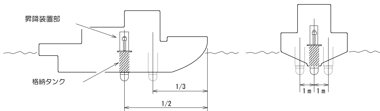
図 1.9 昇降装置部の取付位置
