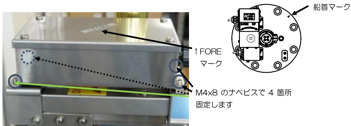
図 1.28 傾斜センサーの取り付け－3
