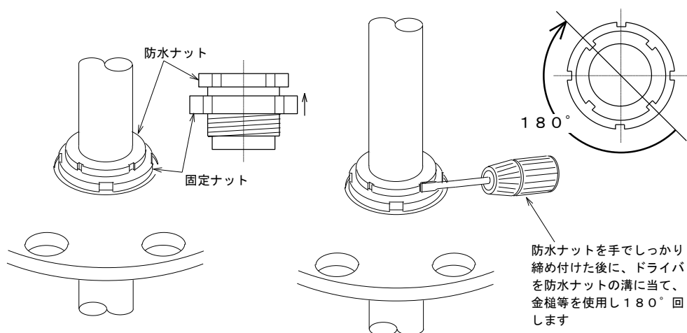
図 1.20 昇降装置部の組立要領-5
