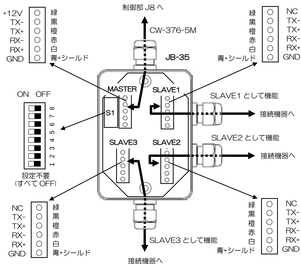
図 1.40 JB-35 の接続
