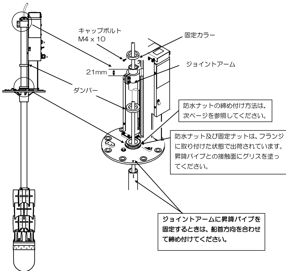
図 1.18 昇降装置部の組立要領-3
