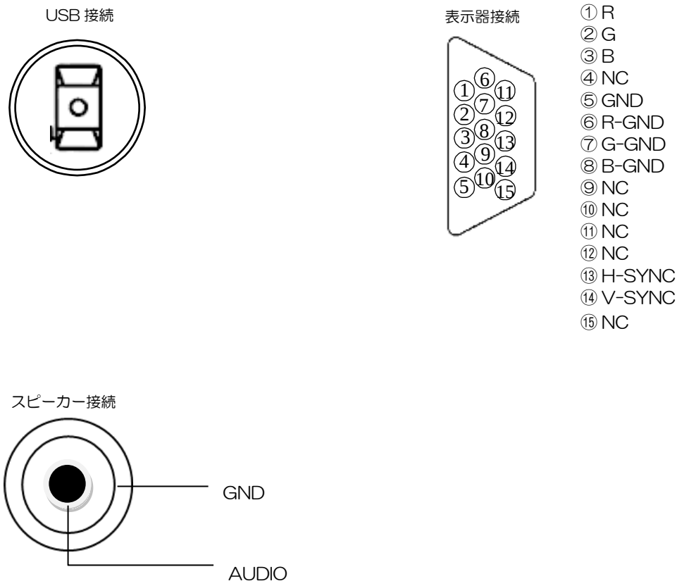
図 1.32 背面コネクタピン配置図-2
