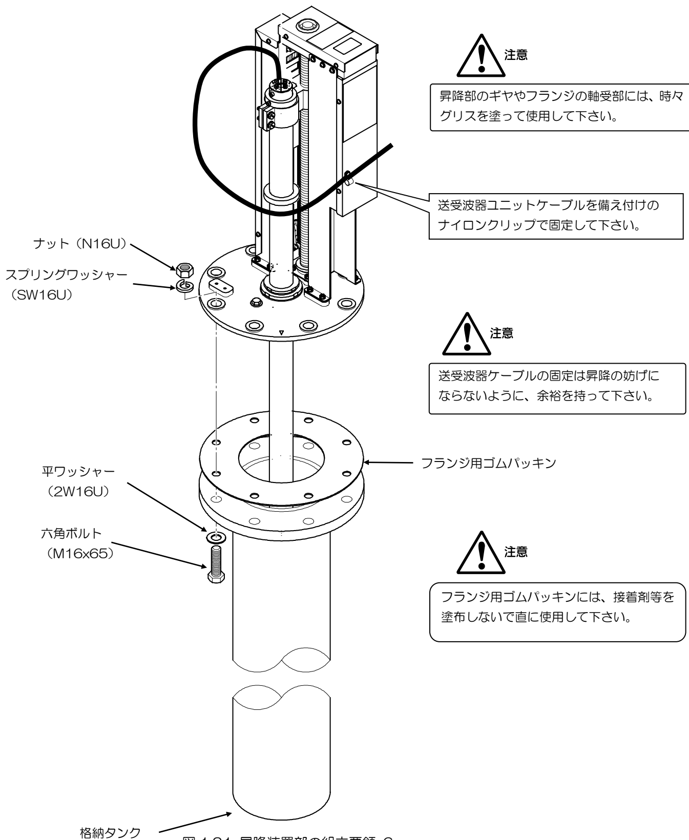
図 1.21 昇降装置部の組立要領-6
