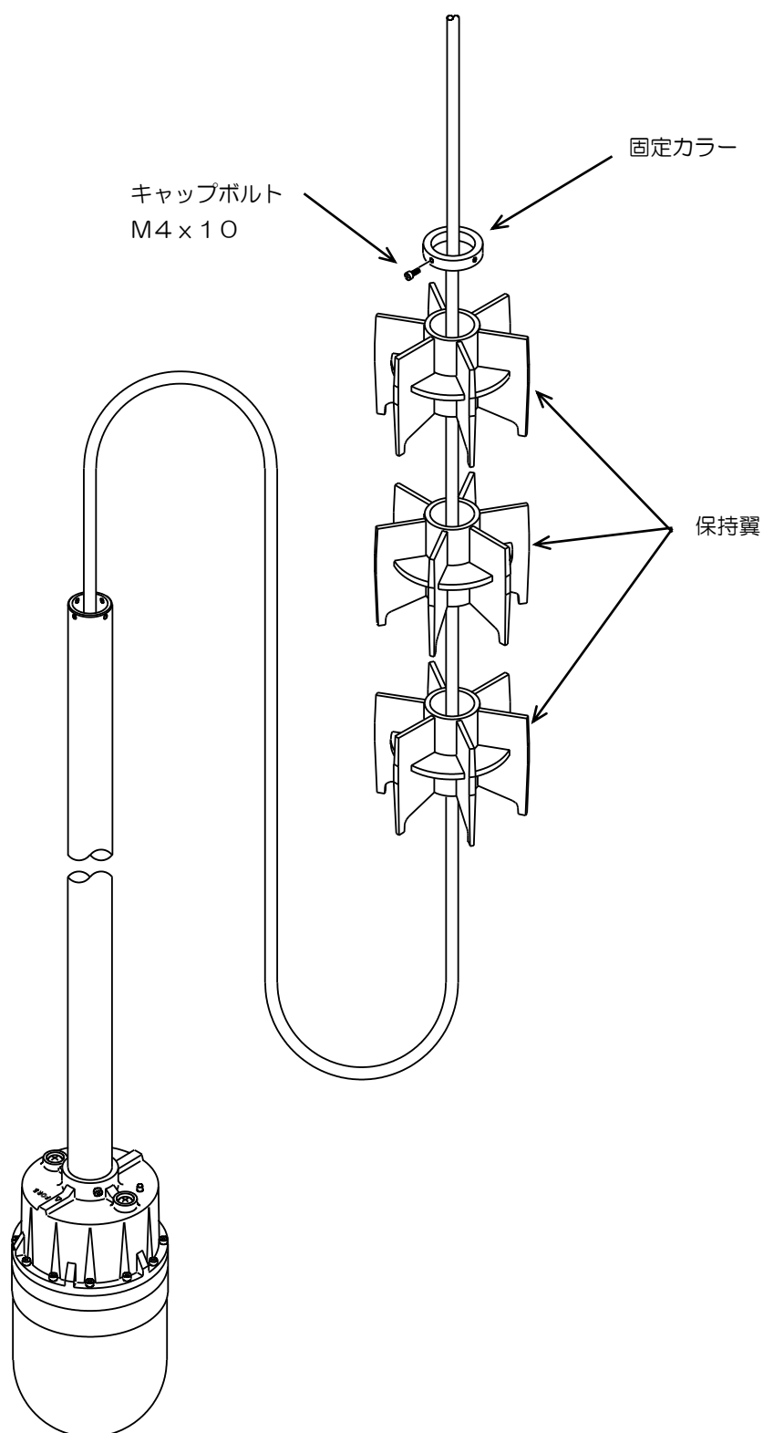
図 1.17 昇降装置部の組立要領-2
