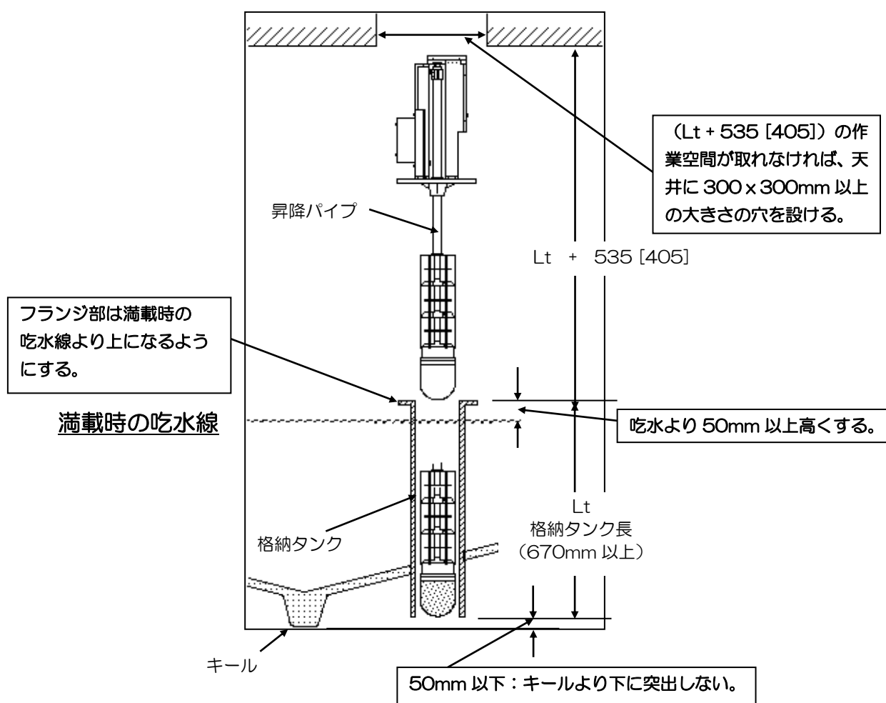
図 1.10 格納タンク設置図
