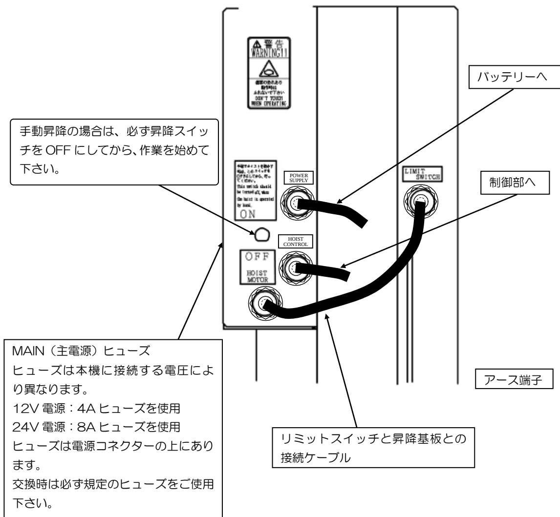
図 1.34 昇降装置ユニット接続部
