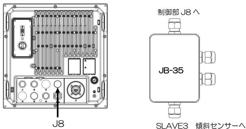
図 1.29 傾斜センサーの取り付け-4
