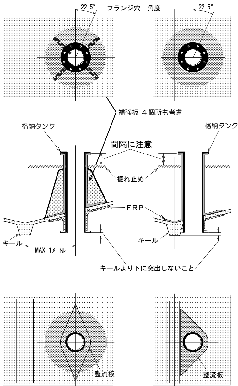
図 1.11 格納タンクの装備
