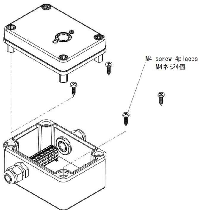
図 1.7 突出警報器の外観図
