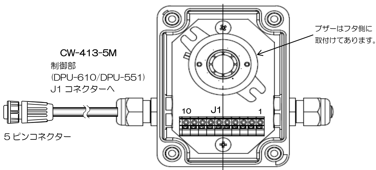
図 1.36 KDS-6000BB/5500BB - 突出警報器 接続図
