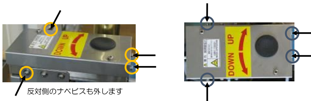
図 1.26 傾斜センサーの取り付け－1
