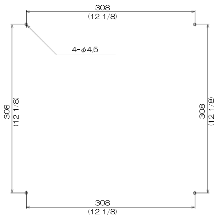
図 1.2 制御部の取付穴加工図
