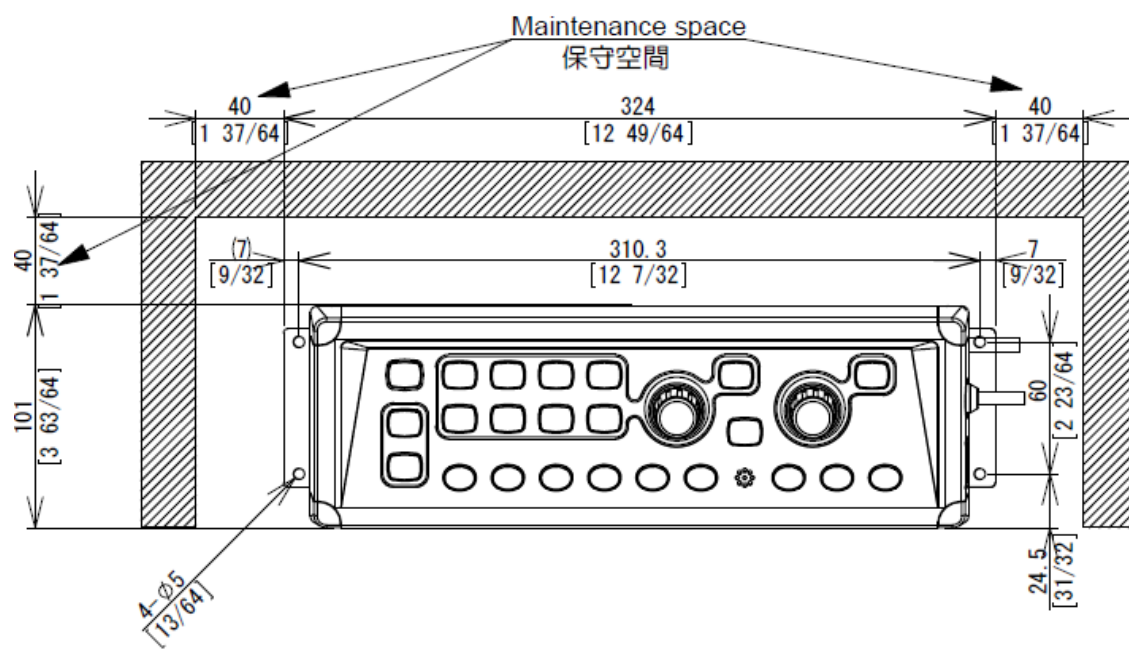
図 1. 4 操作部の卓上取付時の保守空間
