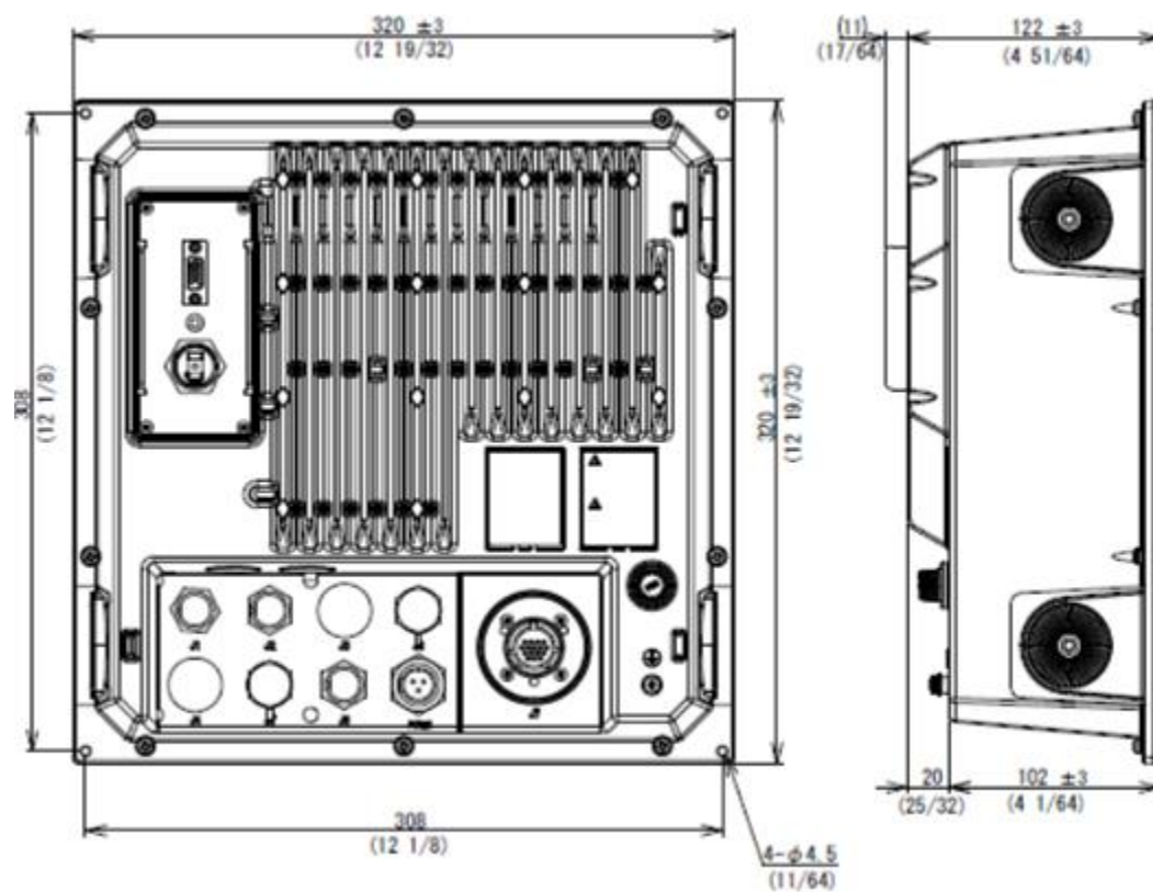
制御部 (DPU-610/DPU-551)
