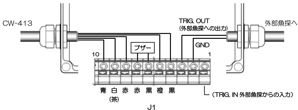
図 1.37 外部魚探 - JB-36 接続図
