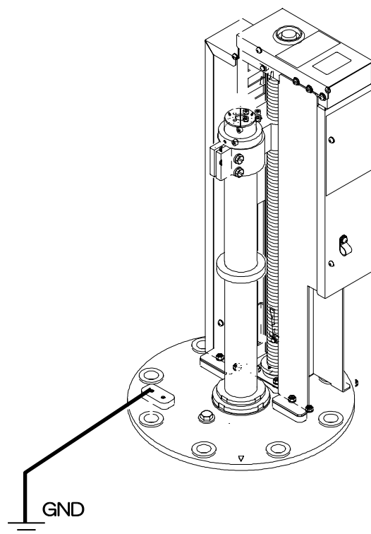
図 1.25 フランジと船体アース接続図
