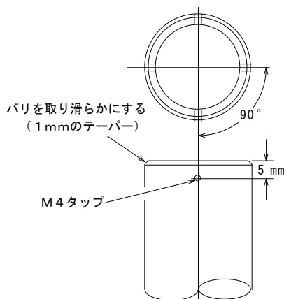
図 1.14 昇降パイプ加工図
