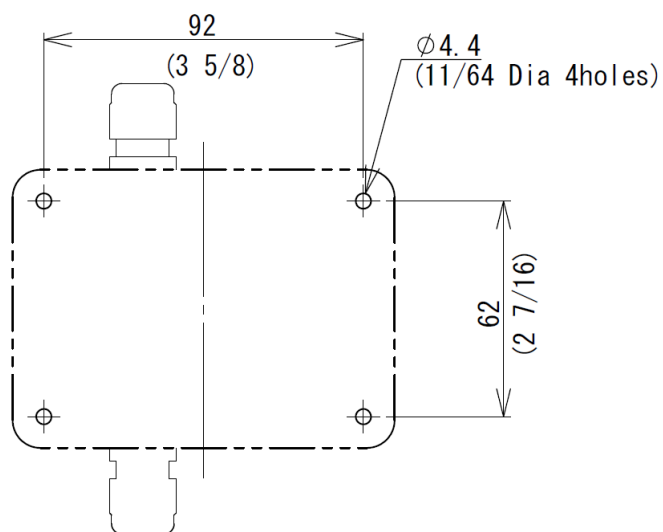
図 1.8 突出警報器の取付穴加工図
