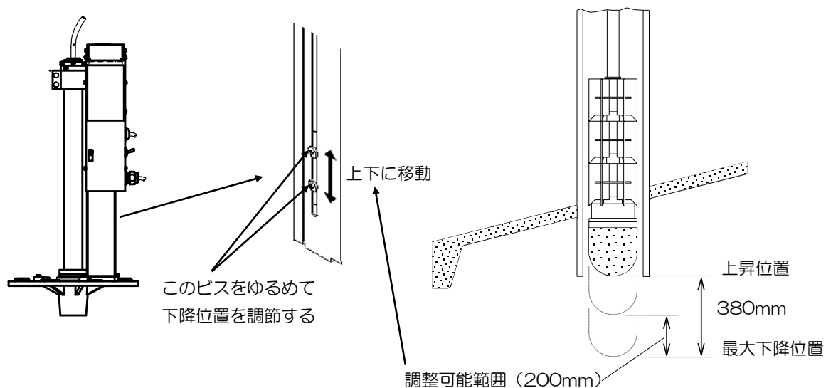
図 1.22 昇降ストロークの調整
