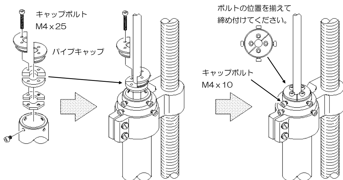
図 1.19 昇降装置部の組立要領-4
