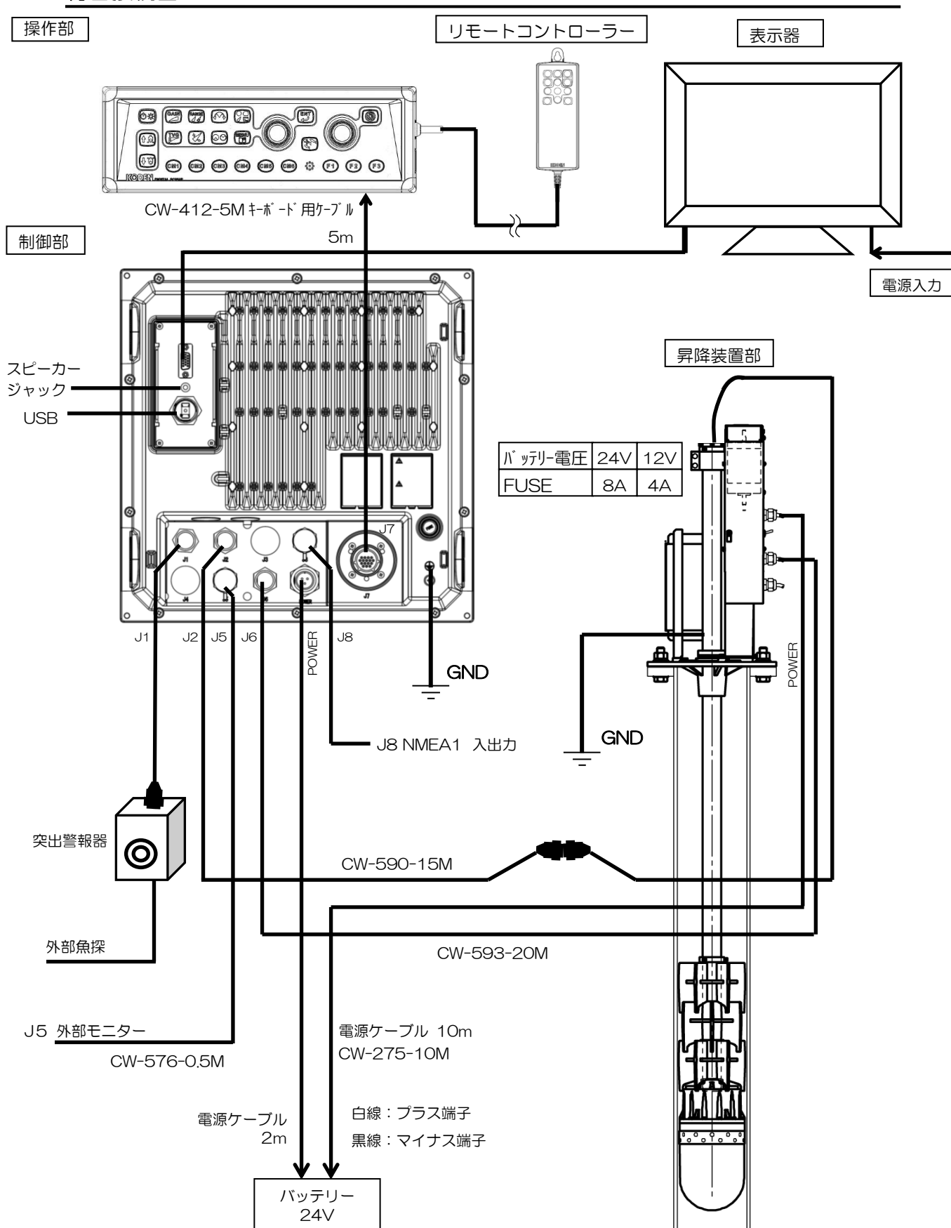
図 1.35 KDS-6000BB/5500BB 接続図
