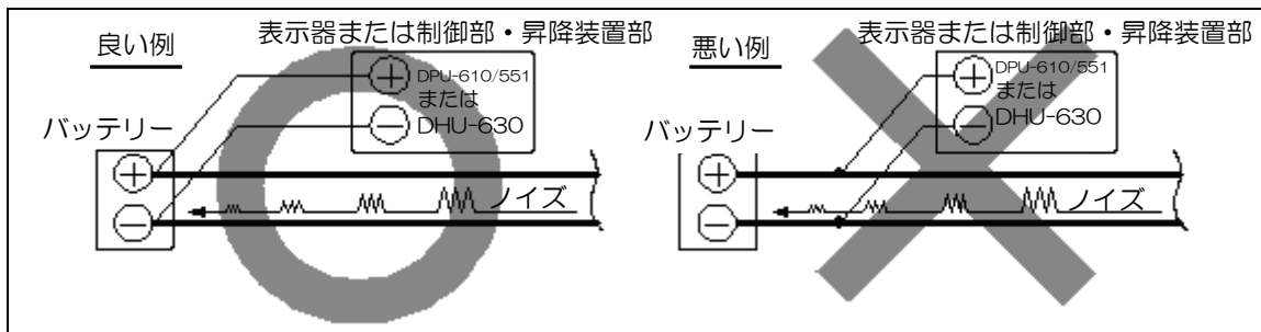
図 1.1 KDS-6000BB/5500BB 電源ラインの接続方法
