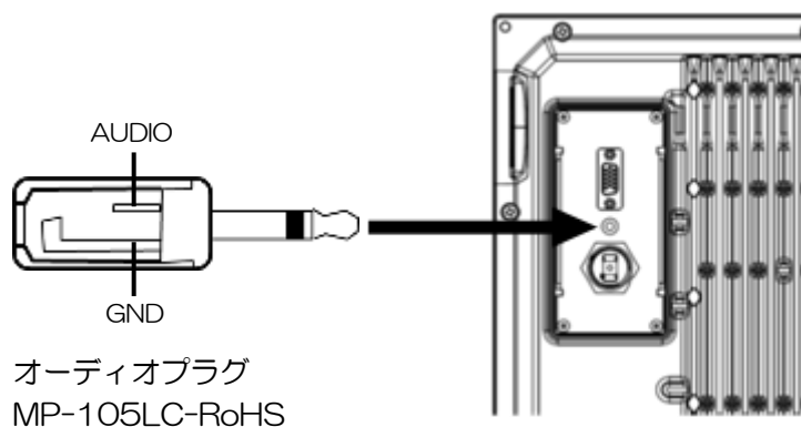
図 1.42 スピーカーの接続
