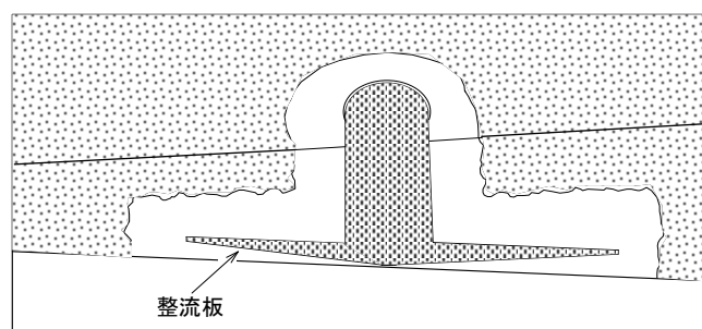
図 1.12 格納タンクの装備例-1
