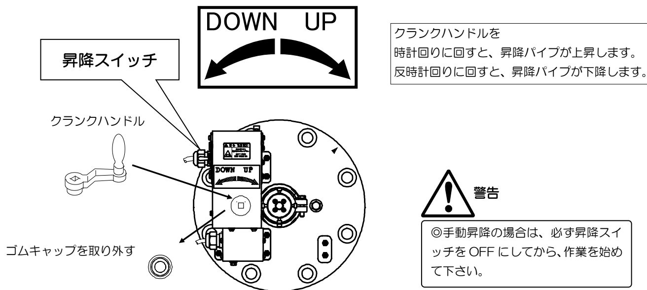
図 1.24 クランクハンドル操作要領
