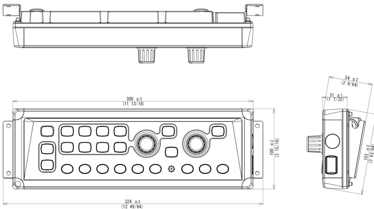
操作部 (DOU-620)
