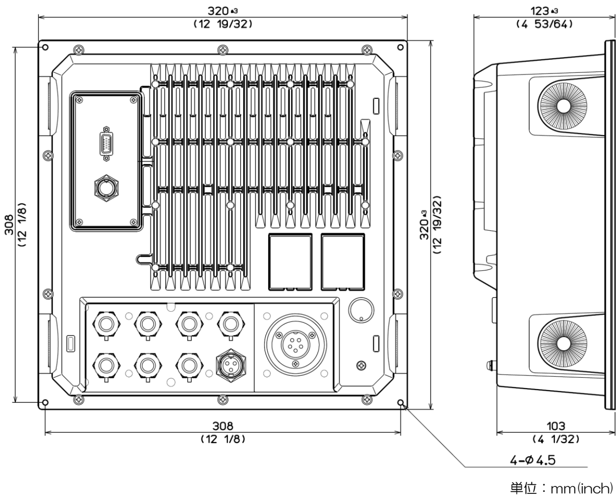
CVS-877D 外觀圖
