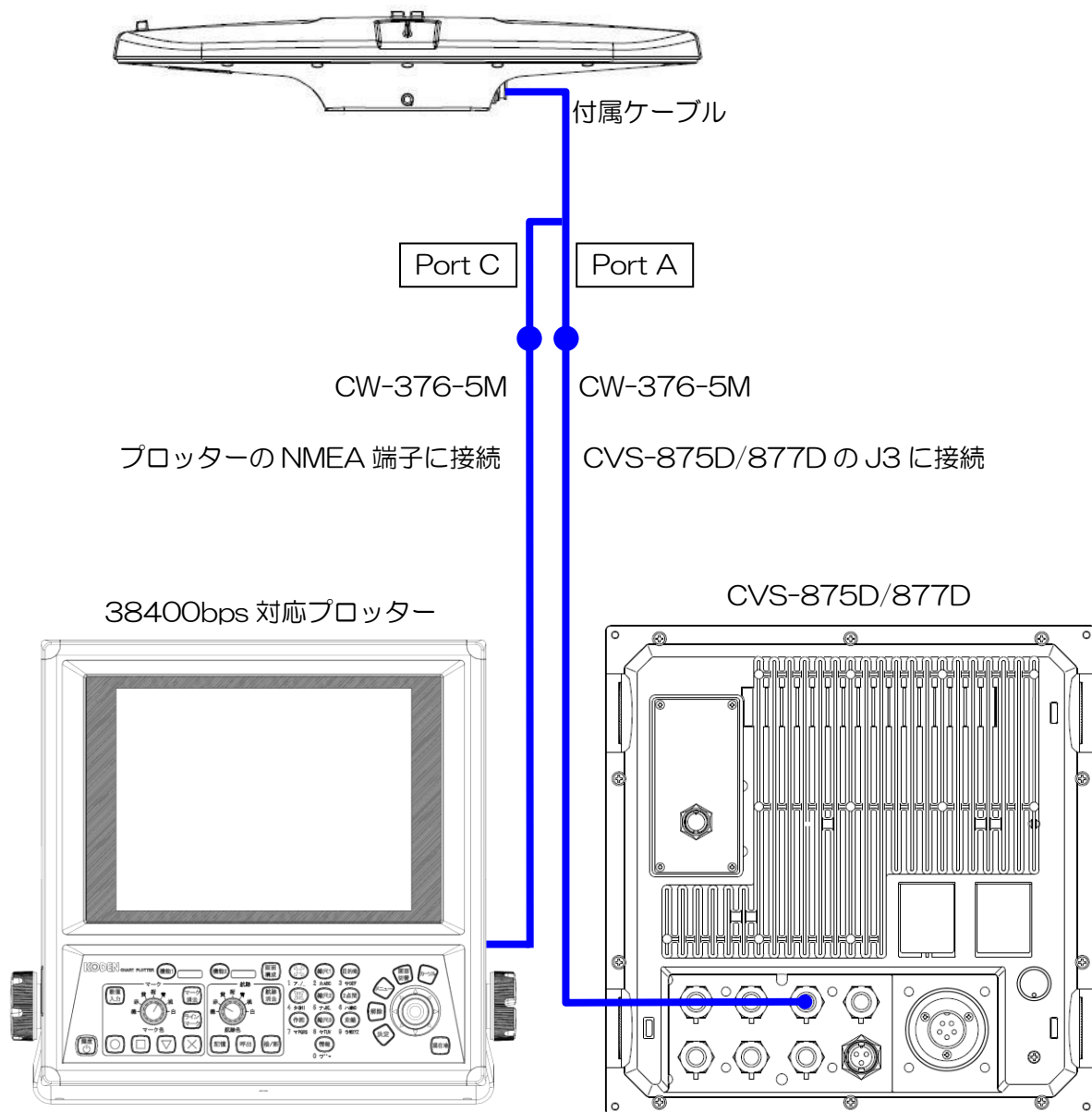
図 1.61 総合接続図 2
