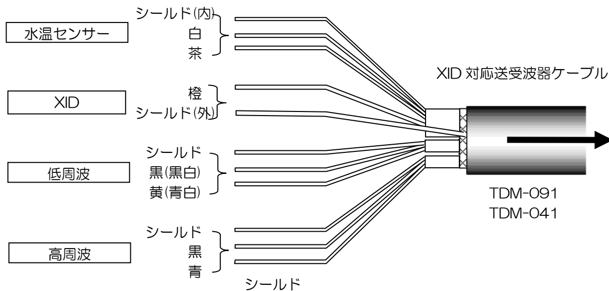
図 1.34 送受波器ケーブル詳細図
