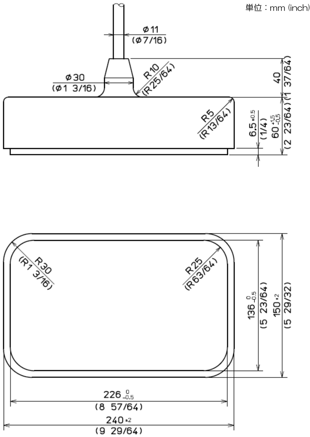
図 1.18 送受波器 TD-754 の外形寸法図
