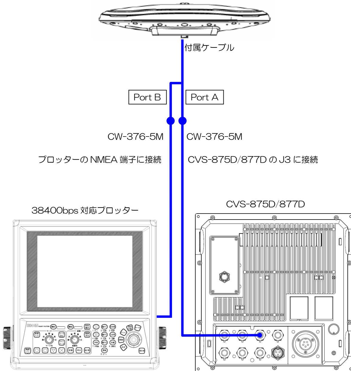
図 1.69 総合接続図 8
