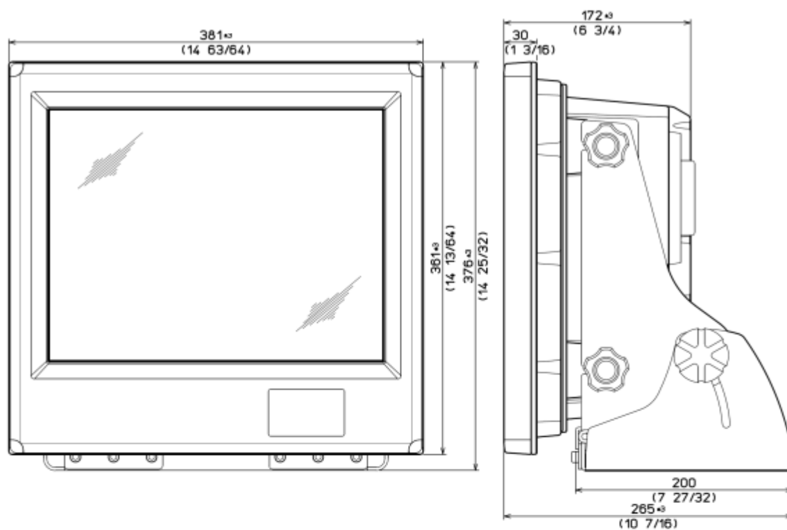
CVS-875D 外觀圖
