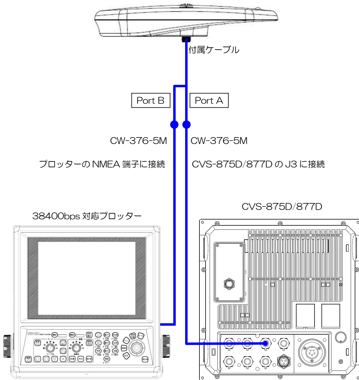
図 1.65 総合接続図 5
