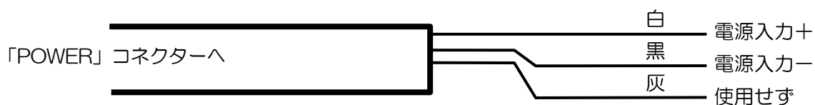
図 1.27 DC 電源ケーブルの接続図
