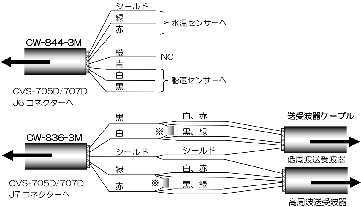
図 1.26 送受波器ケーブル接続図
