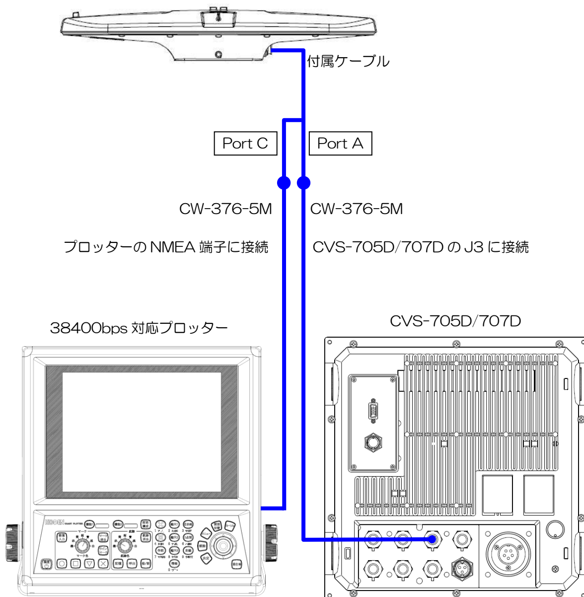
図 1.48 総合接続図 2
