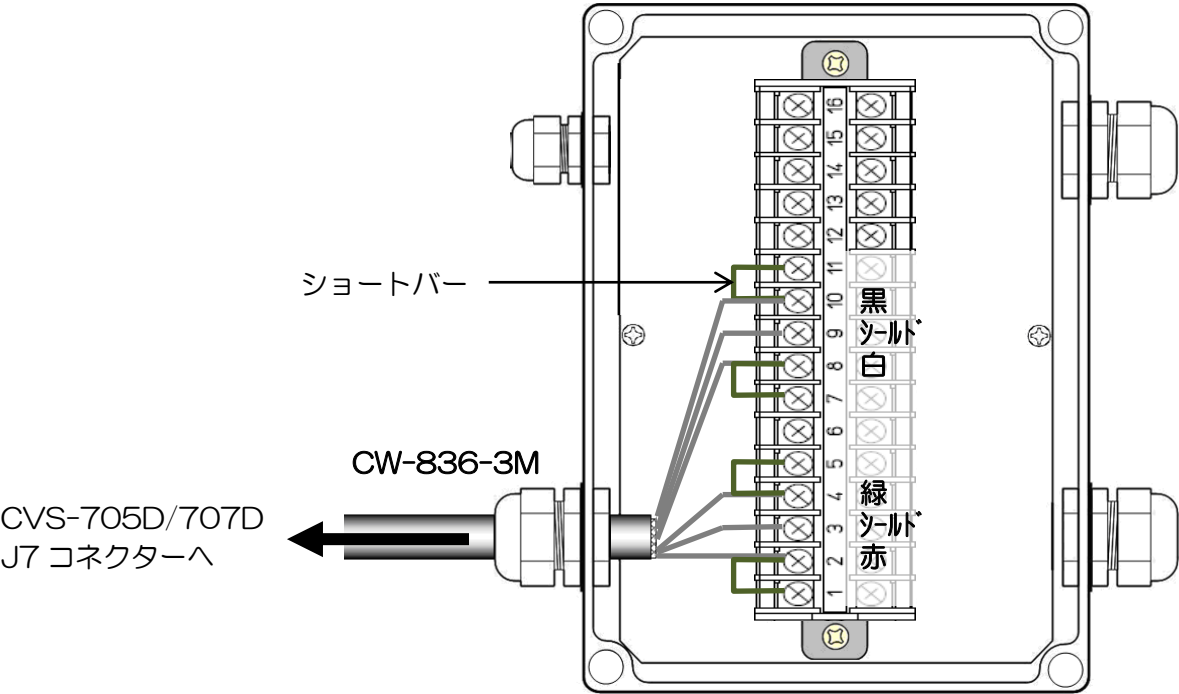
図 1.27 CVS-705D/707D – ジャンクションボックス接続図
