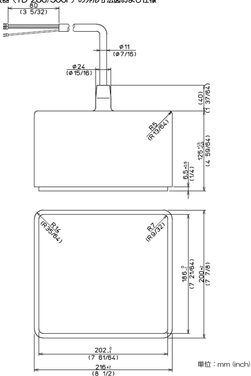
図 1.17 送受波器 (TD-286/TD-506F) の外形寸法図 送受波器 (TD-286/TD-506F) の仕様
