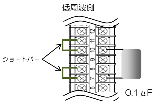
図 1.33 ジャンクションボックス — コンデンサー接続図
