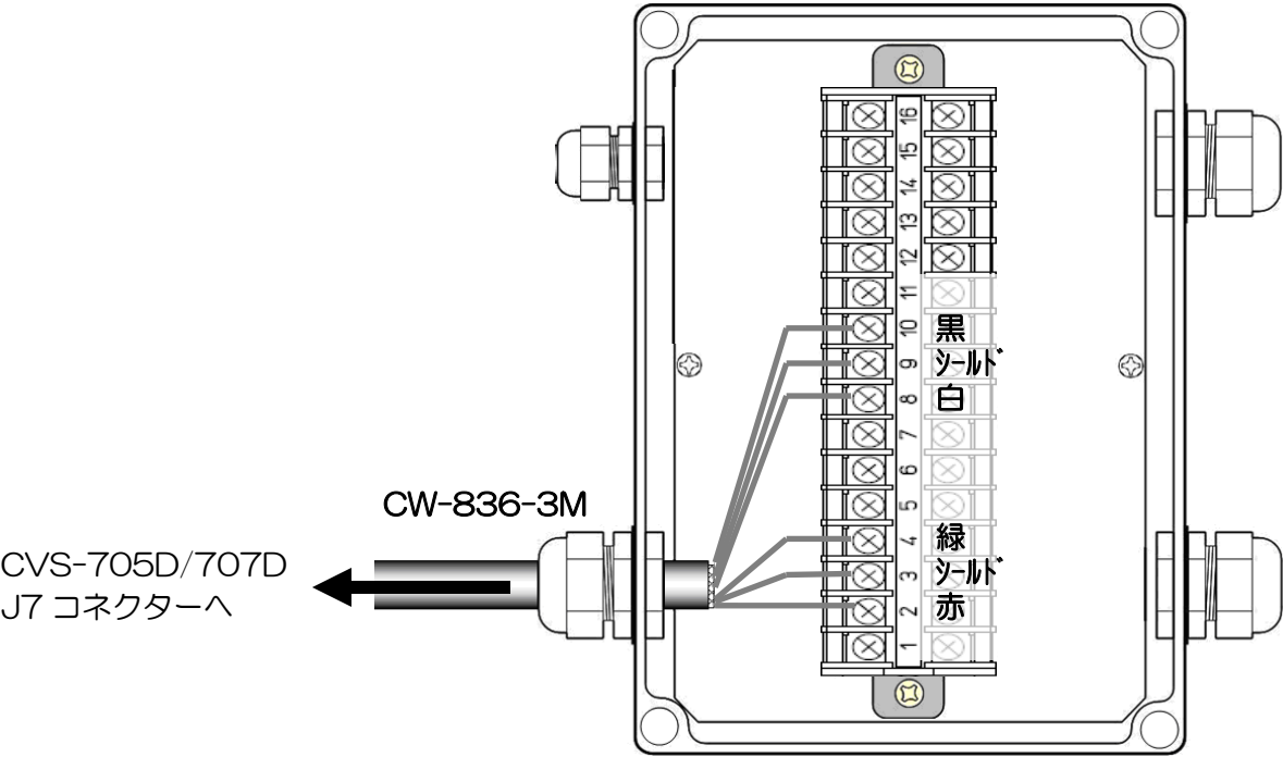
図 1.35 CVS-705D/707D – ジャンクションボックス接続図
