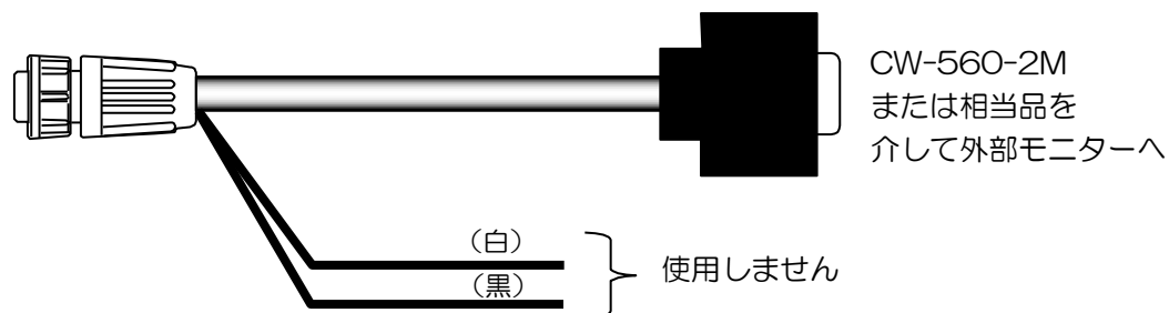
図 1.42 外部モニター接続図-1
