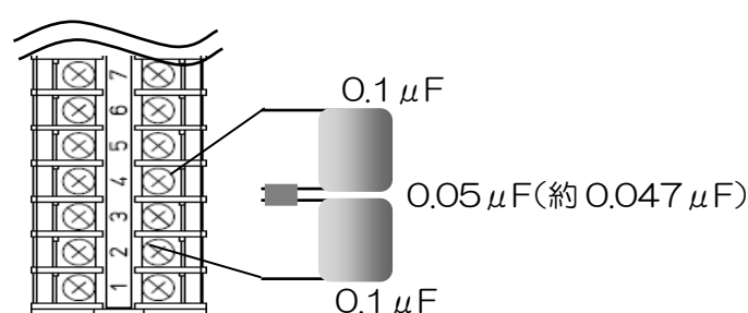
図 1.37 ジャンクションボックス — コンデンサ接続図
