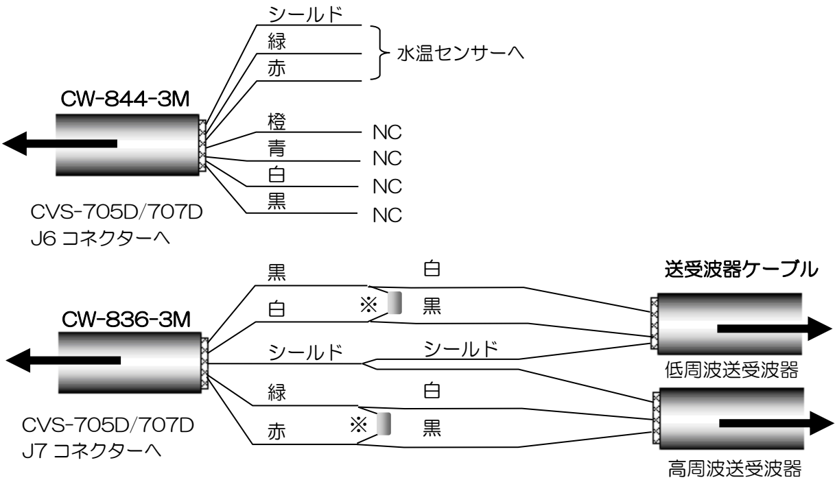
図 1.34 送受波器ケーブル接続図
