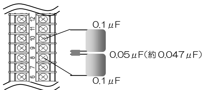
図 1.39 ジャンクションボックス — コンデンサー接続図
