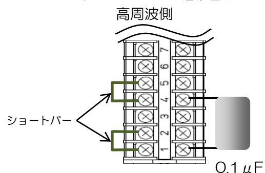
図 1.29 ジャンクションボックス — コンデンサー接続図
