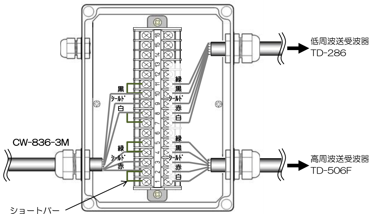
図 1.28 ジャンクションボックス — 送受波器接続図
