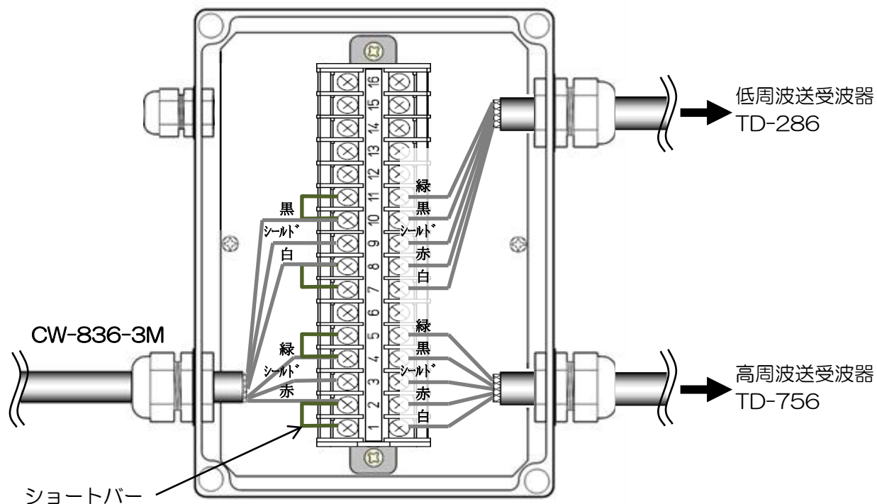
図 1.30 ジャンクションボックス — 送受波器接続図
