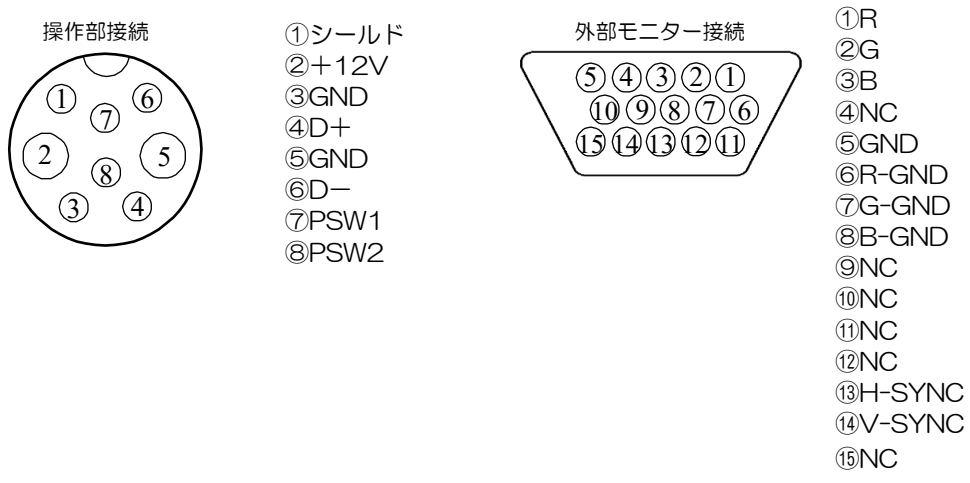
図 1.24 背面コネクタピン配置図-2
