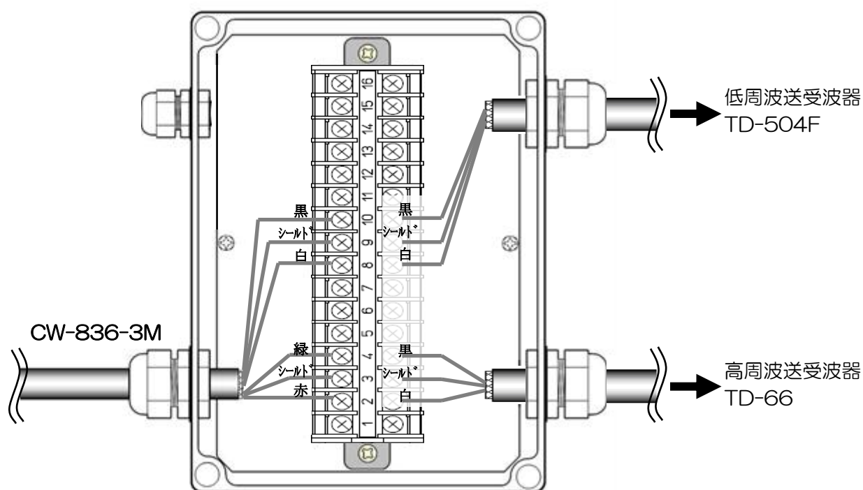
図 1.38 ジャンクションボックス — 送受波器接続図
