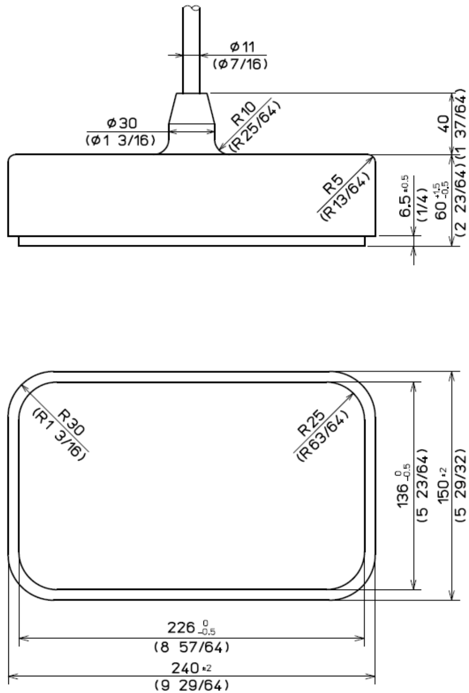
図 1.21 送受波器 TD-754 の外形寸法図
