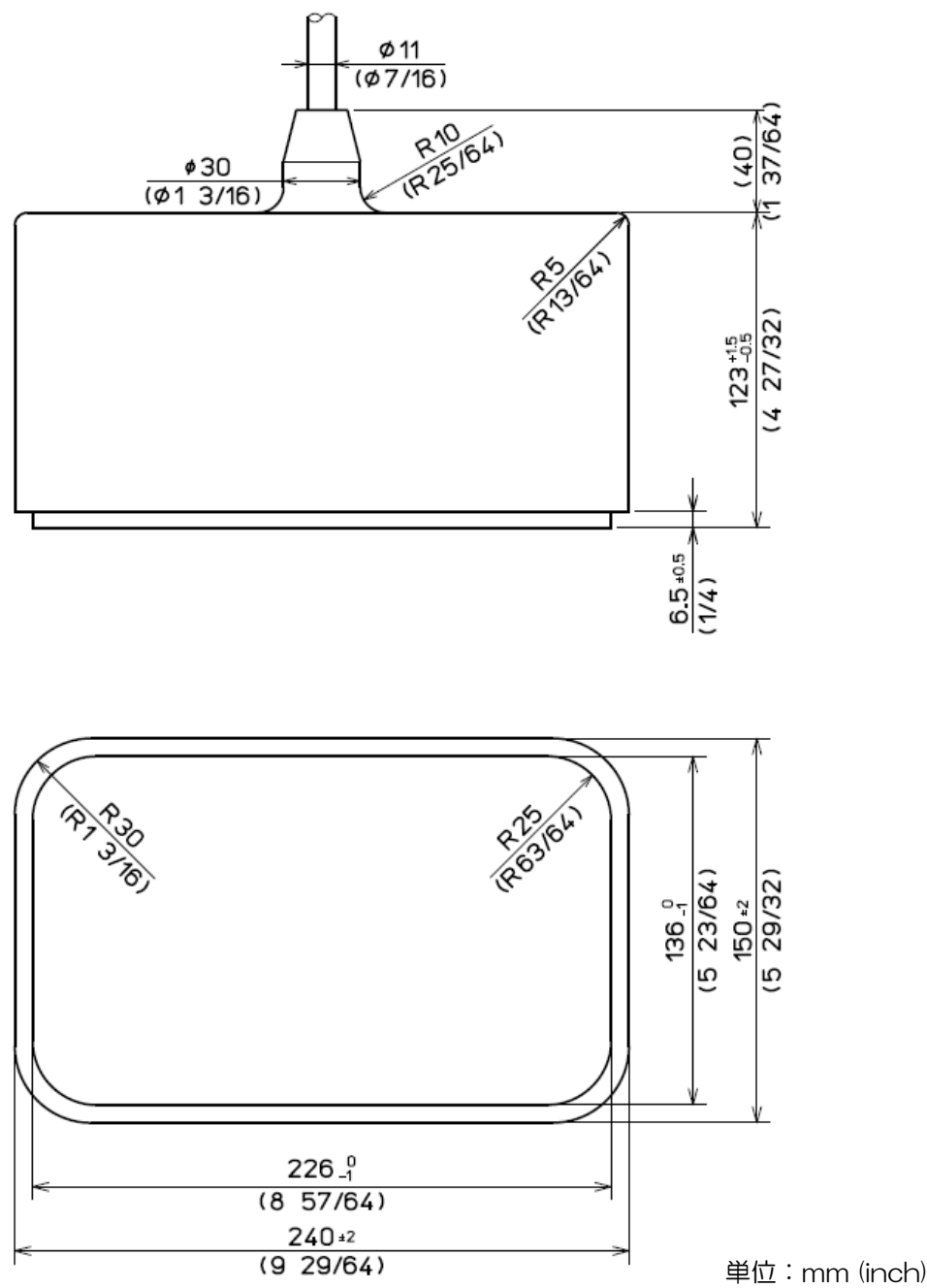
図 1.20 送受波器（TD-284/TD-284A/TD-404T/TD-504T/TD-504F）の外形寸法図
