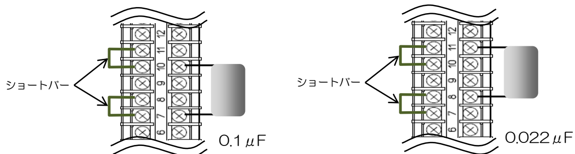
図 1.31 ジャンクションボックス — コンデンサー接続図
