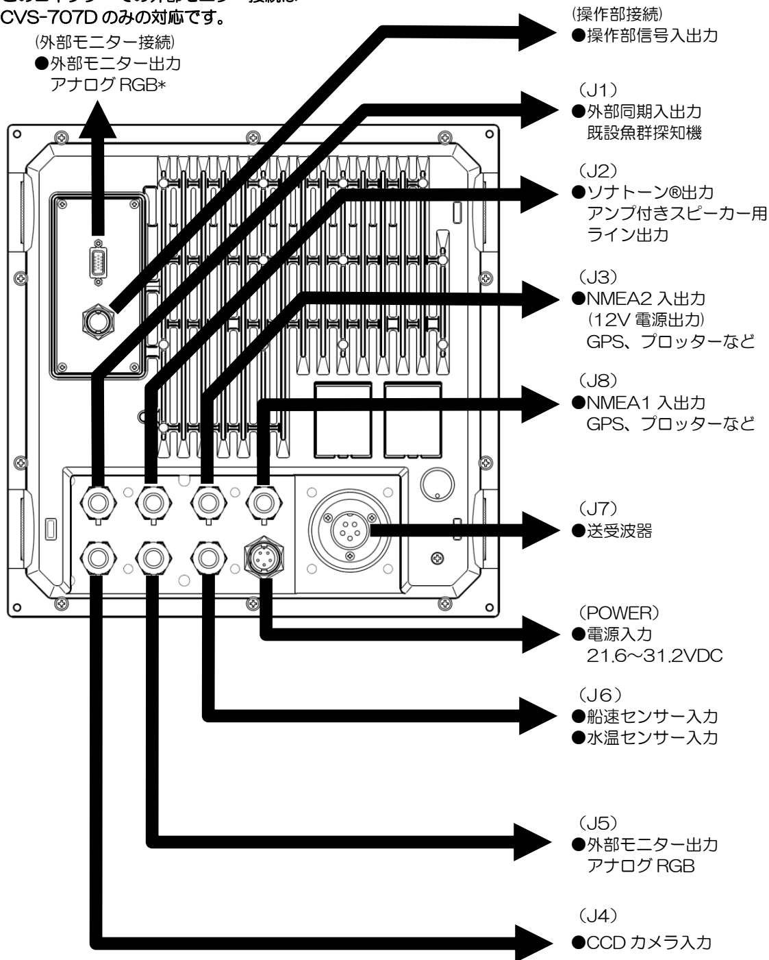
図 1.22 ケーブル接続図
