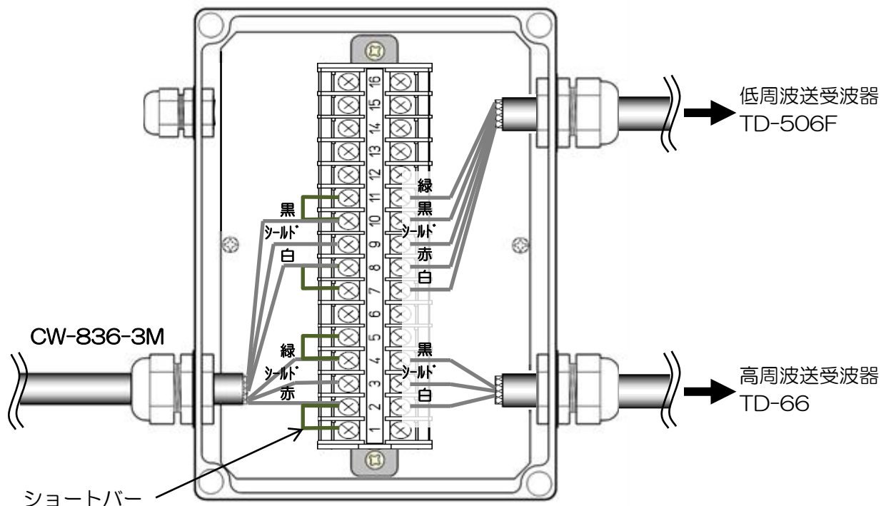
図 1.32 ジャンクションボックス — 送受波器接続図
