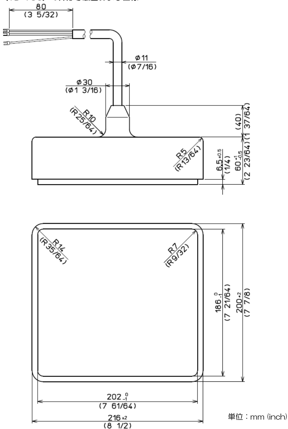
図 1.18 送受波器 TD-756 の外形寸法図
