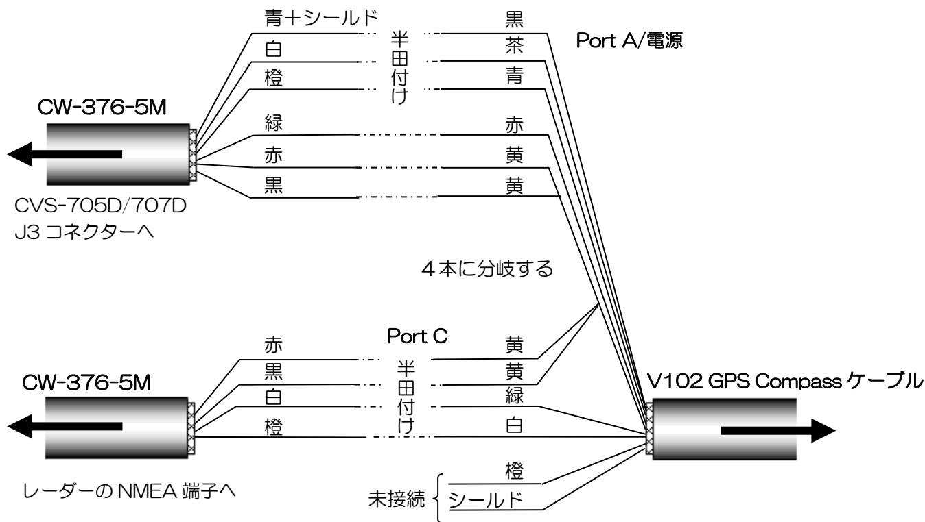
図 1.46 V102 GPS Compass ケーブル接続図
