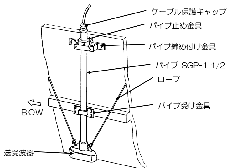
図 1.15 送受波器舷側装備図
