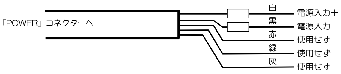
図 1.25 DC 電源ケーブルの接続図
