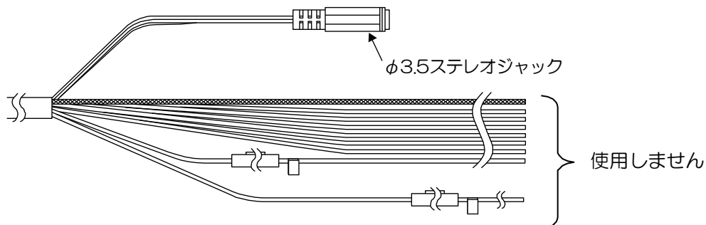
図 1.41 ソナトーン®用外部スピーカー接続図
