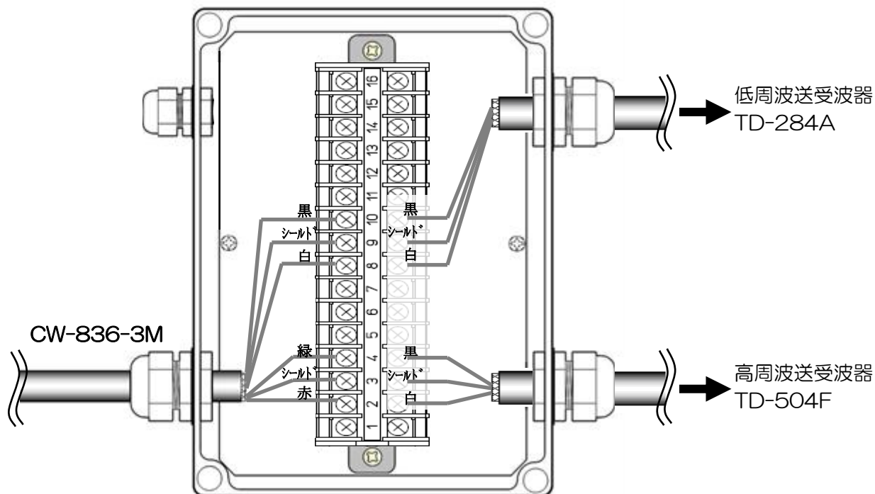
図 1.36 ジャンクションボックス — 送受波器接続図
